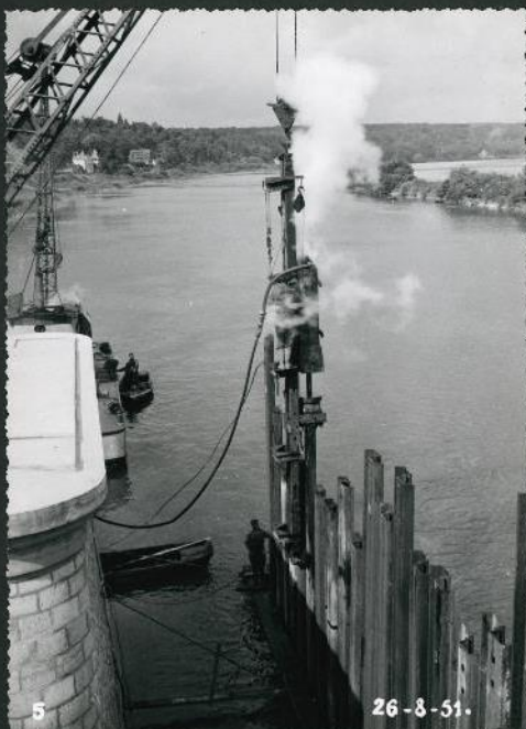
MOULIN À VAPEUR en ACTION
