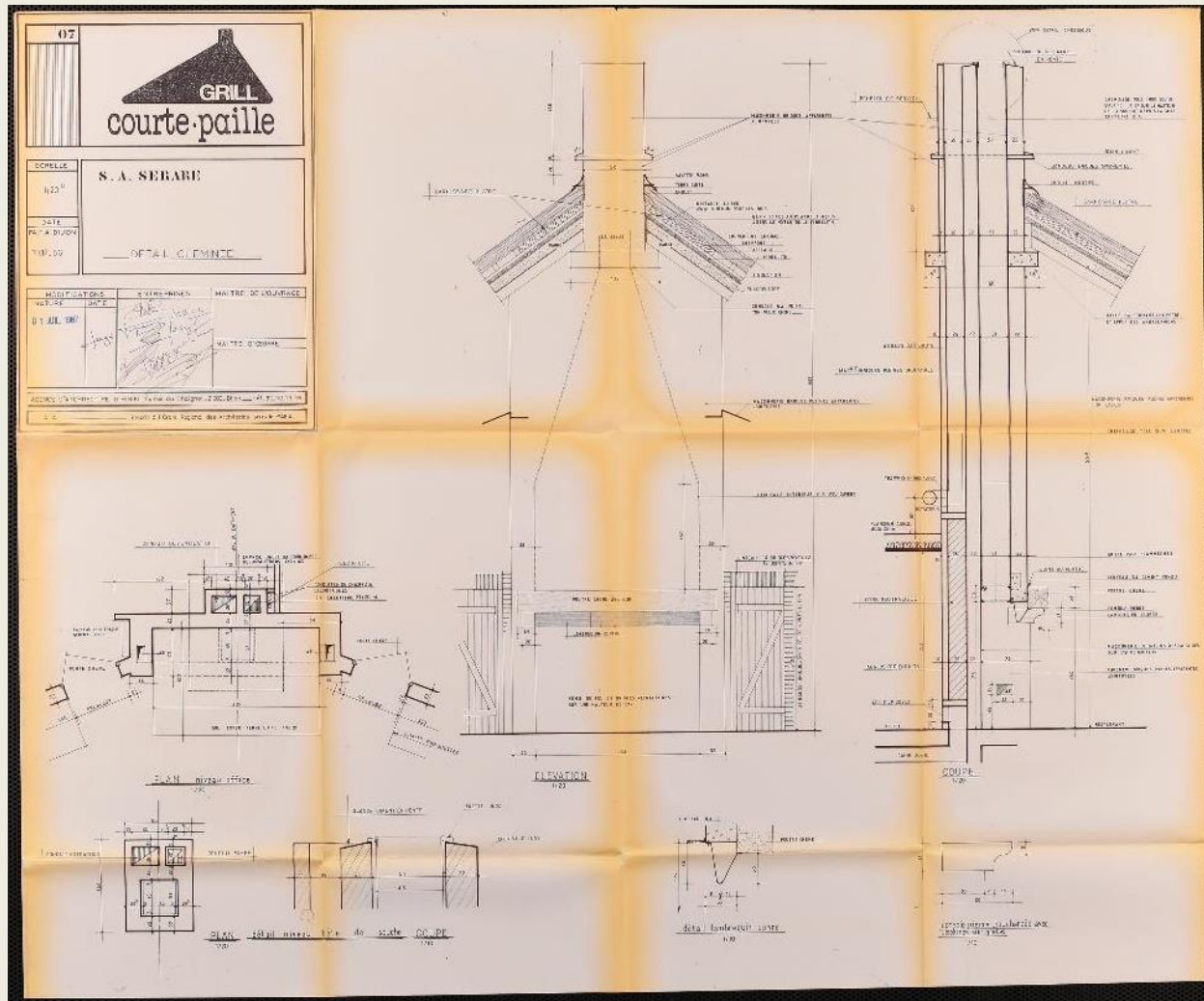
371 J_001 – Plan du Courte-paille de Lognes, détail de la cheminée, 1986-1987
