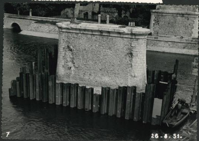
BATARDEAU de la PILE de DROITE, TERMINÉ
